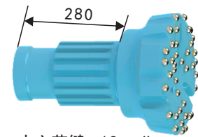
十六花键 16 splines
